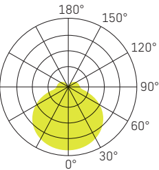
LICHTVERTEILUNGSKURVE
