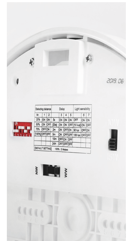
Einstellmöglichkeiten Sensorleuchte
